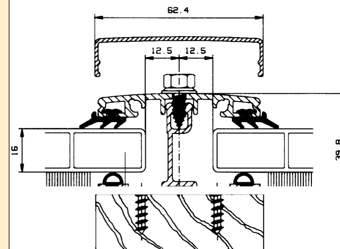
Komplettsprosse 16 inkl. Dichtungsprofilen, Sprossenprofilen, gelocht, pressblank Profilbreite ca. 6 cm
