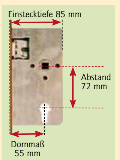
3. Dornmaß
